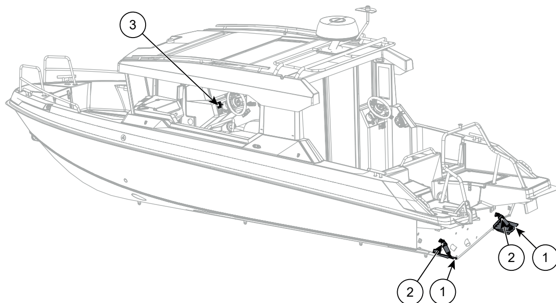
Figur 5.6 Placering av trimsystemets komponenter
