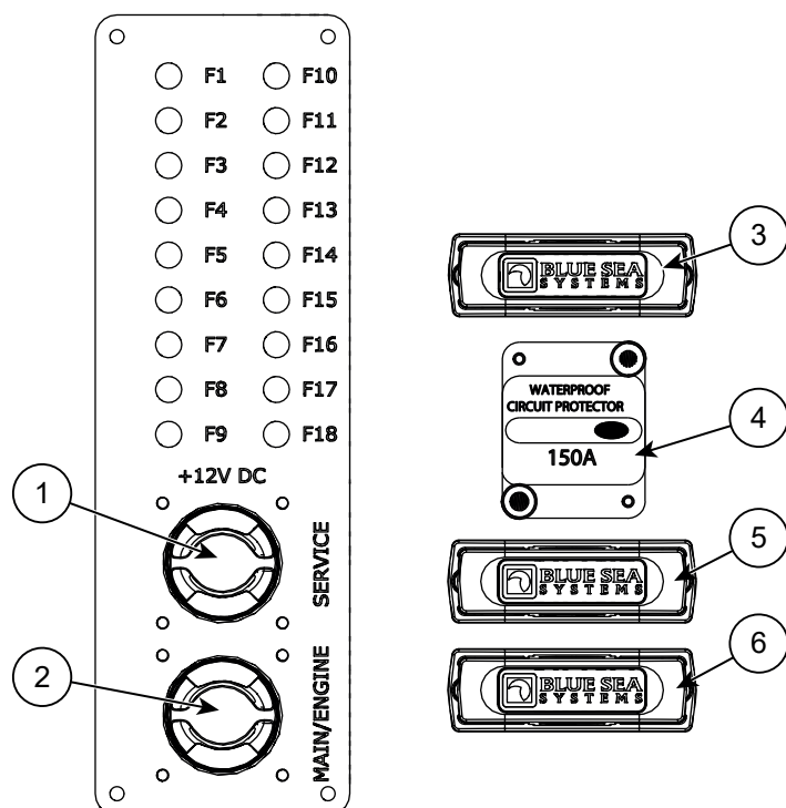
Figur 8.1 Buster Magnum Cabin - huvudströmbrytare och säkringspanel
