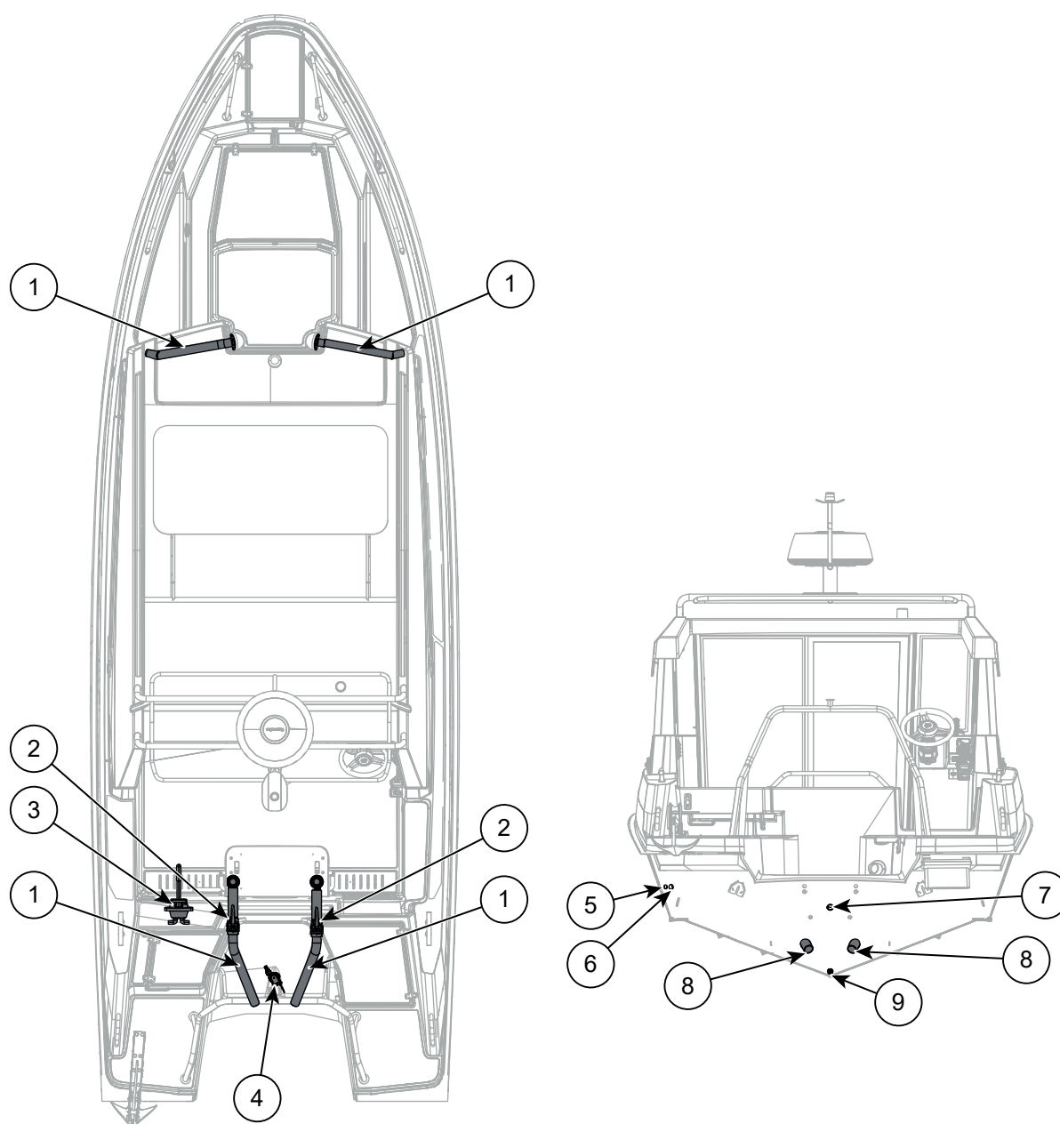
Figur 9.1 Buster Magnum Cabin - dräneringsutrustning
