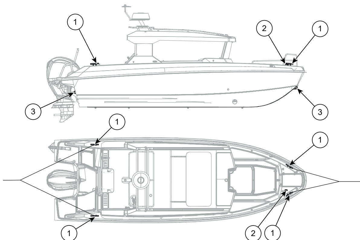
Figur 5.7 Buster Magnum Cabin förtöjnings- och bogseringspunkter
