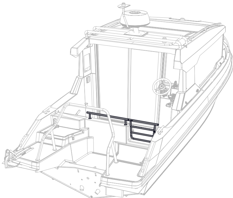
Figur 4.2 Ombordstigningsgrind på Buster Magnum Cabin
